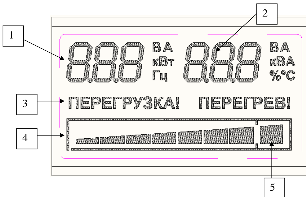
Рисунок 3 – ЖК-дисплей
