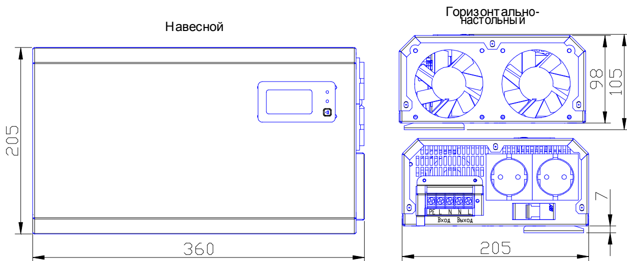
Рисунок 1.2. – Габаритные размеры стабилизатора Штиль и рекомендованные варианты установки
