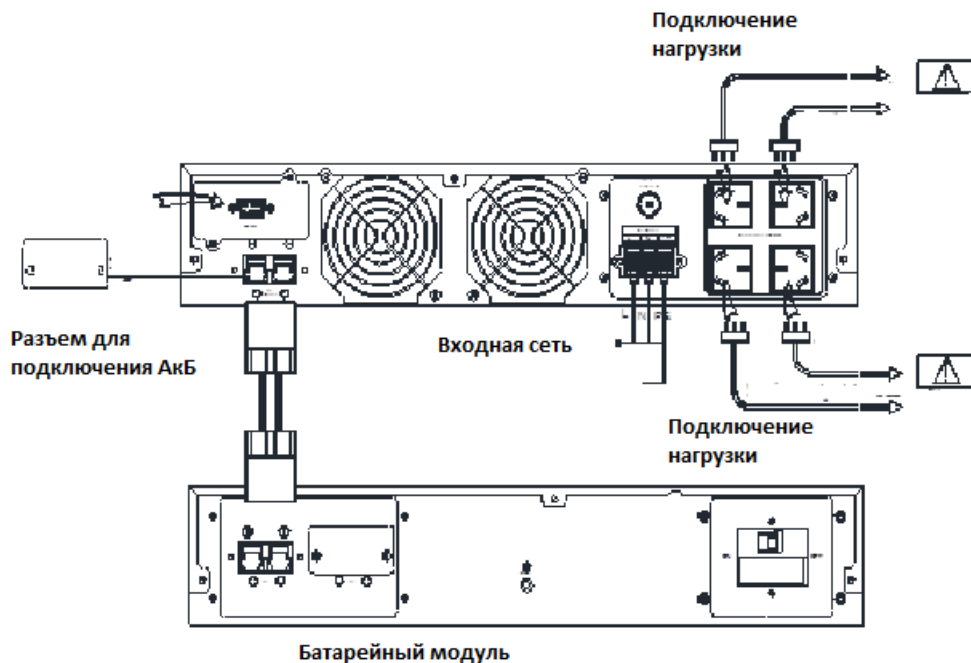
Рис. 3-3 Схема подключения ИБП 1102-1103 (L)
