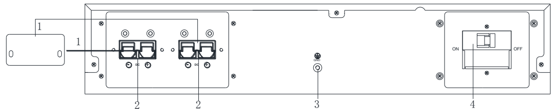
рис.2-4 Задняя панель батарейного модуля
