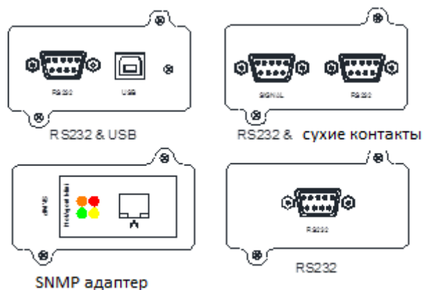
Рис. 2-7 Коммуникационные интерфейсы
