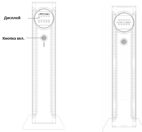
ИБП и батарейный модуль в настольном исполнении
