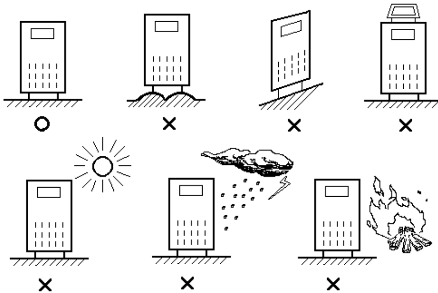
Рис. 3-1 Предупреждения при установке ИБП
