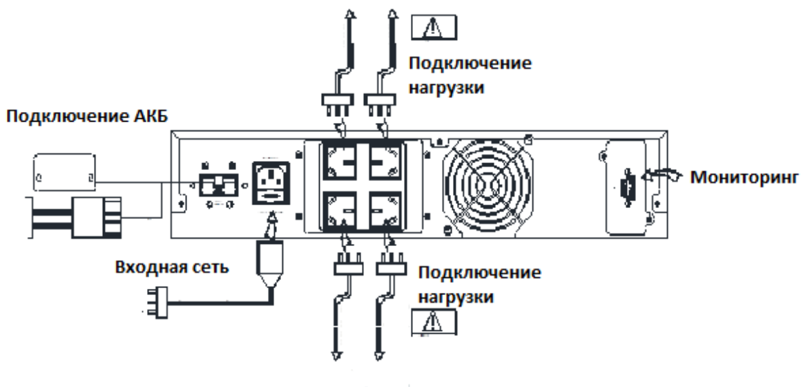
Рис. 3-2 схема подключения ИБП HR1101HS (L)
