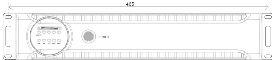
ИБП для установки в телекоммуникационную стойку
